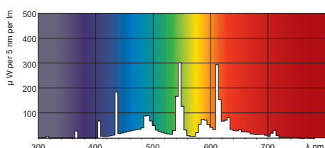
Lightcolor TL-D de Luxe /940
