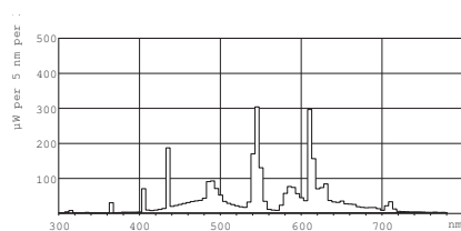
Lightcolor TL-D de Luxe /940
