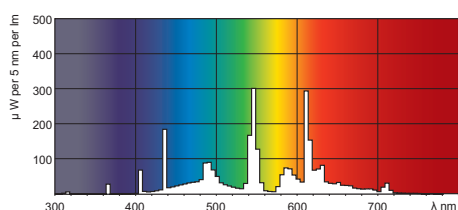
Lightcolor TL-D de Luxe /940
