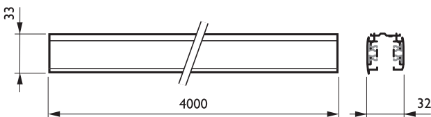
RCS750 5C6 L4000 BK
