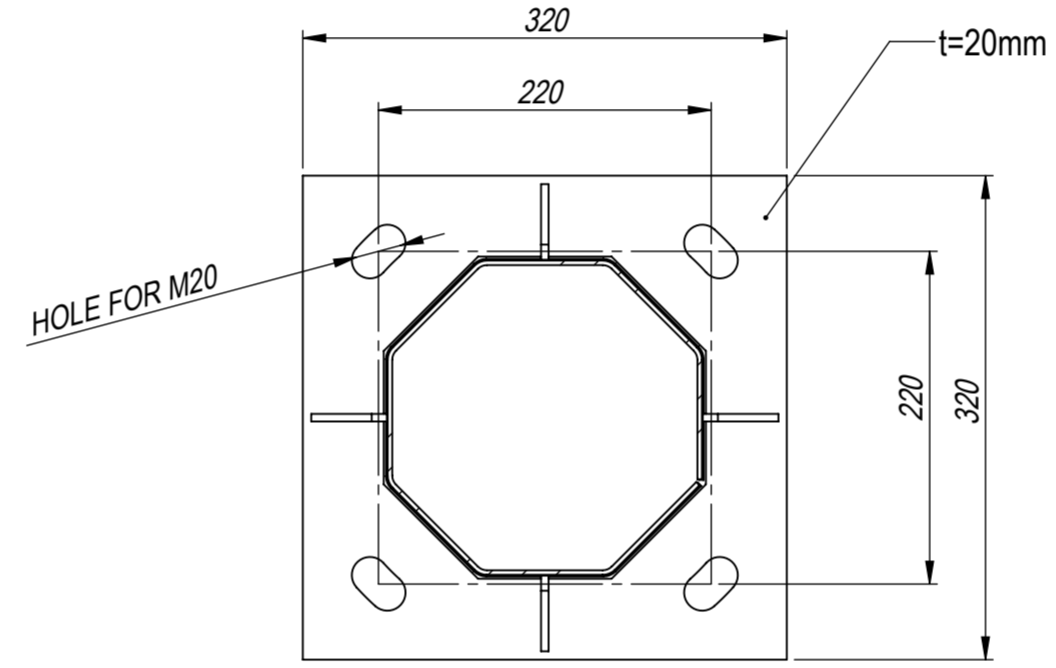
A-A (1:5)
