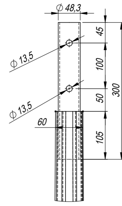
DETAIL C SCALE: 1/5
