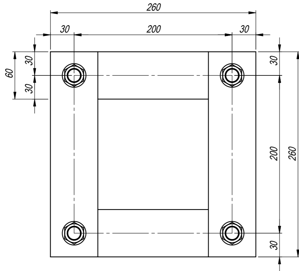
A-A (1:3)
