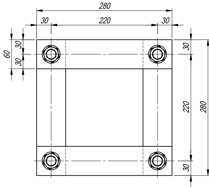
A-A (1 : 4)
